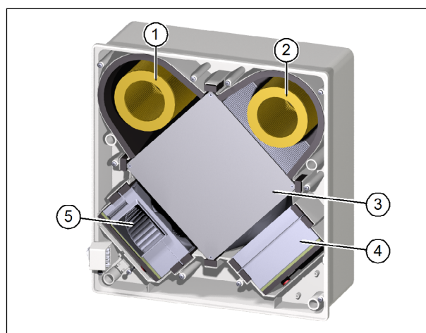
Abb. 8: Komponenten für den Luftaustausch
